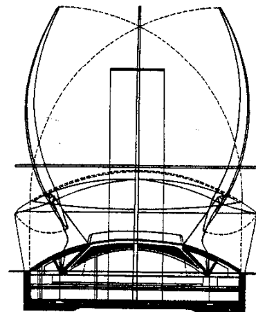
Corte
