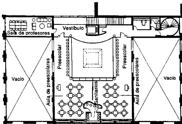
Planta superior
