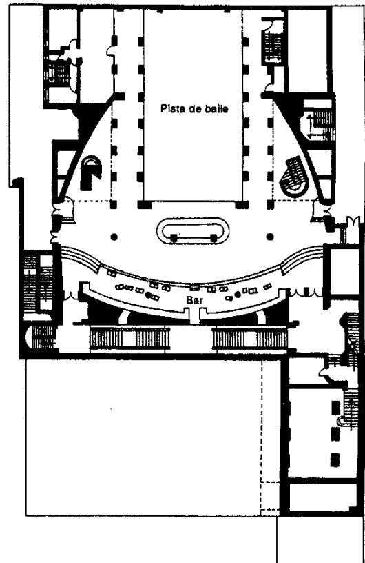
Planta segunda
