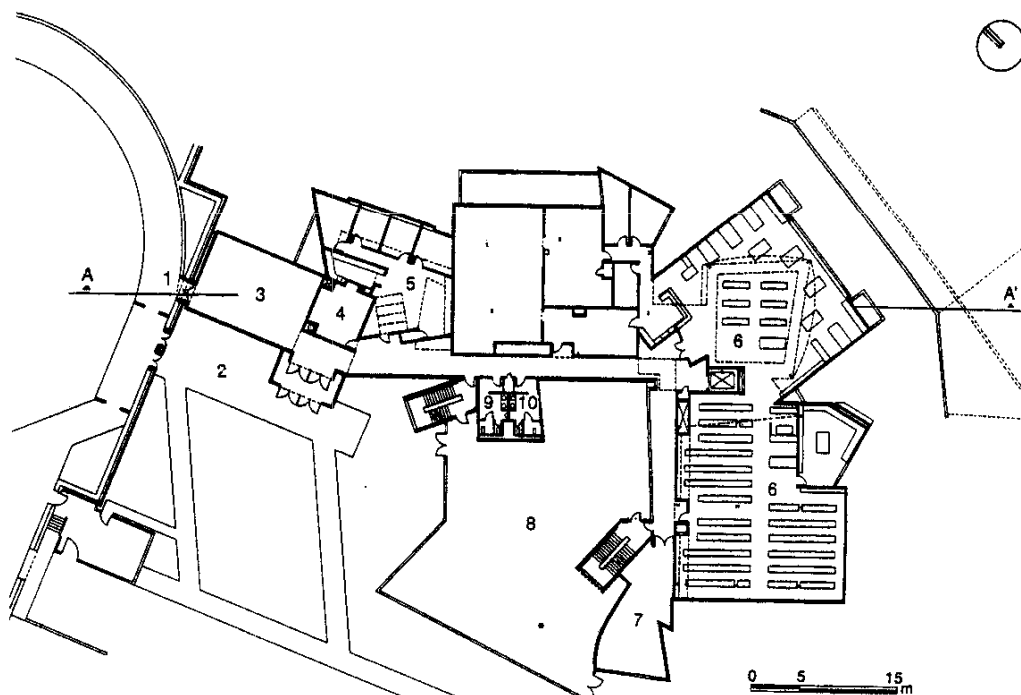
Planta general
