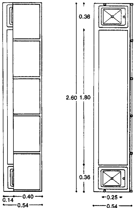
Planta nivel 1
