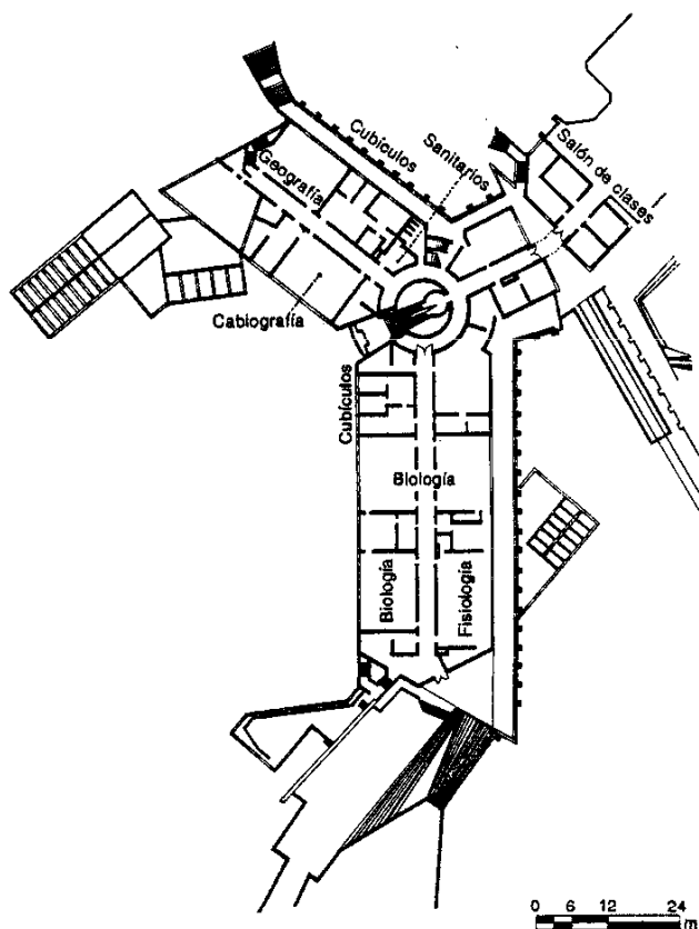
Planta alta
