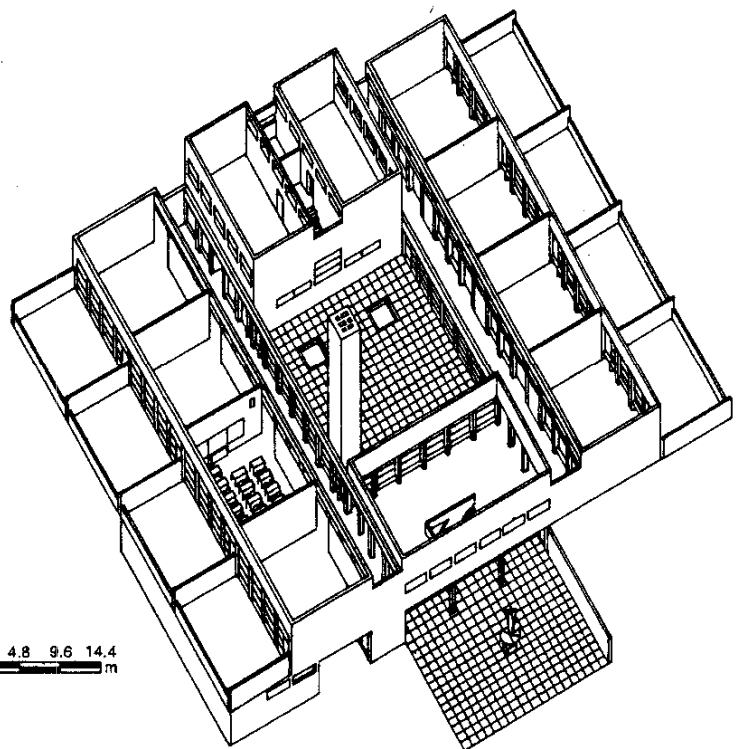
Axonométrico
