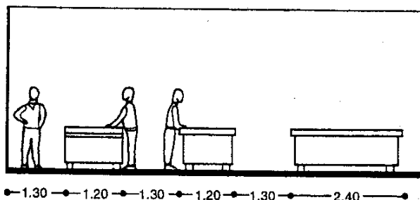
Espacios de trabajo, taller de carpintería
