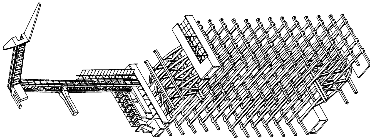
Axonométrico
