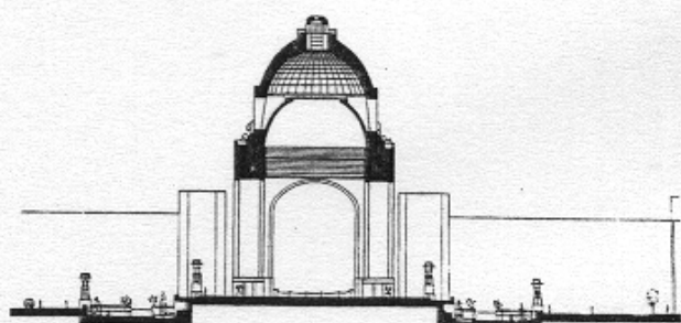
Corte transversal
