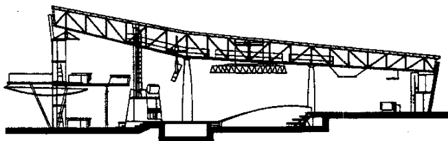
Cortes longitudinales
