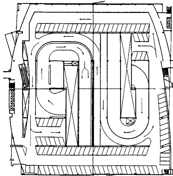
Planta nivel azotea
