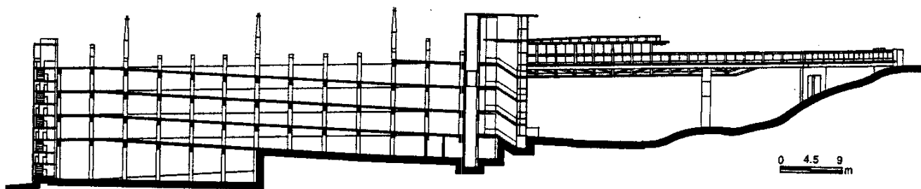
Corte general
