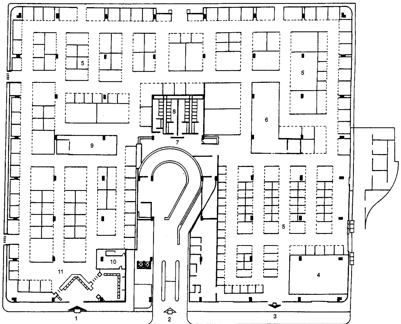
Planta general
