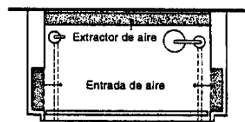
Bancos con almacén incluido
