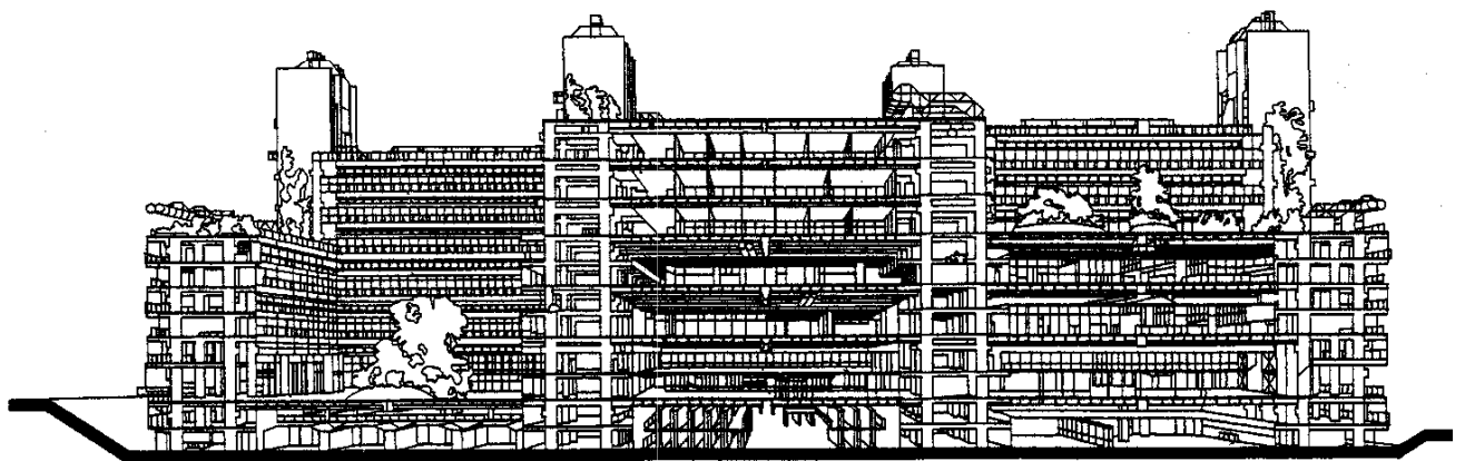
Corte perspectivado
