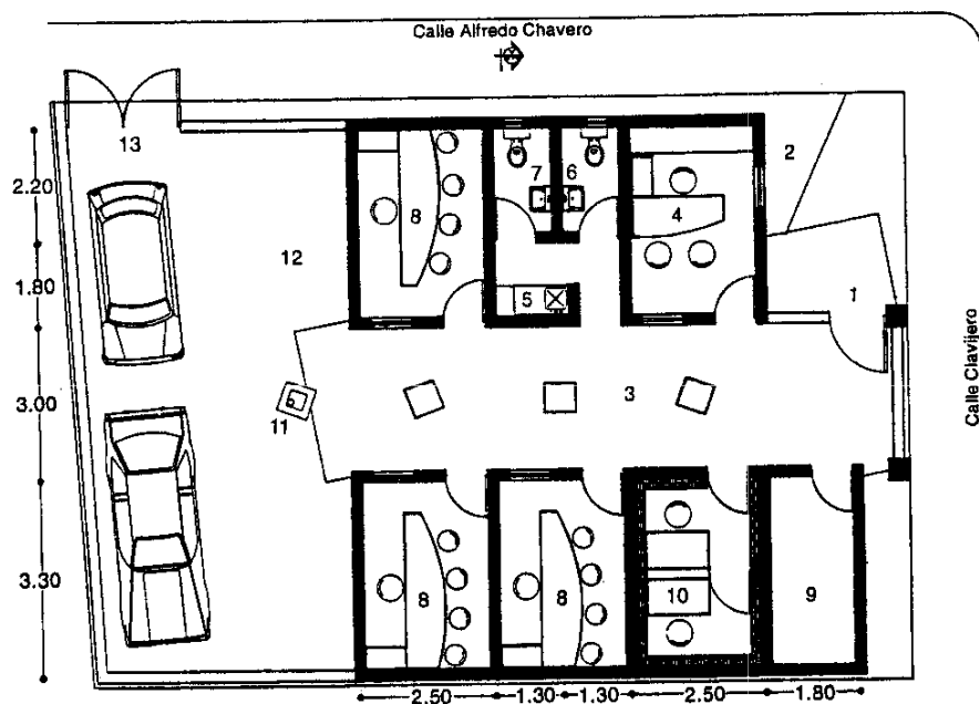
Planta baja
