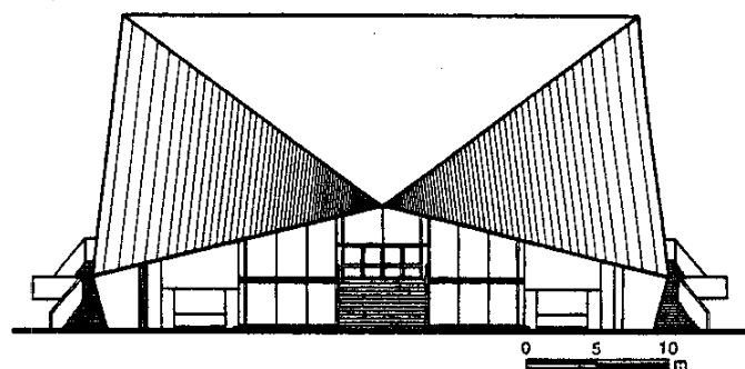
Fachada noroeste
