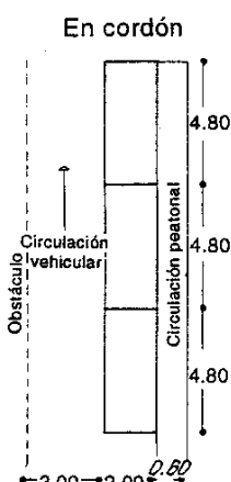
En cordón
