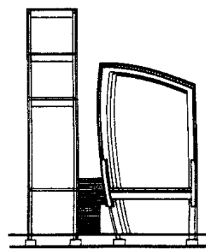
Corte
