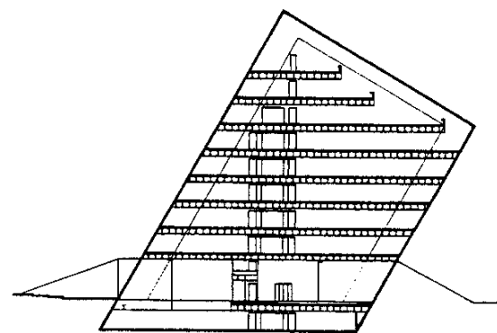
Corte longitudinal
