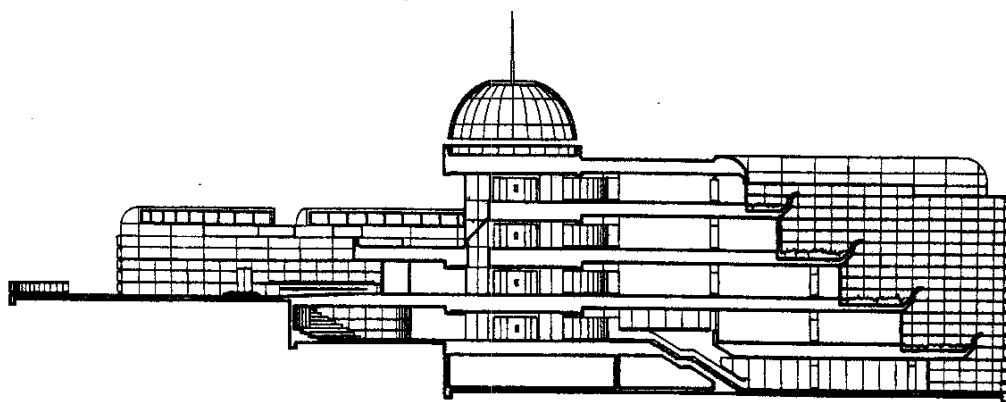
Corte norte-sur
