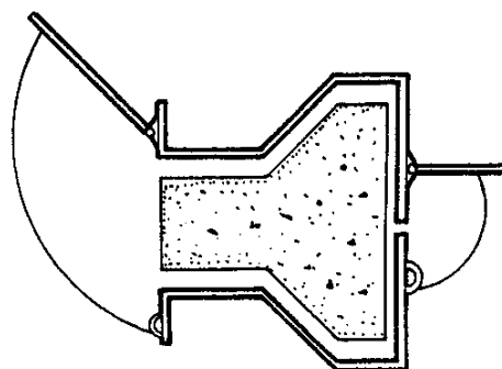
Encofrar
