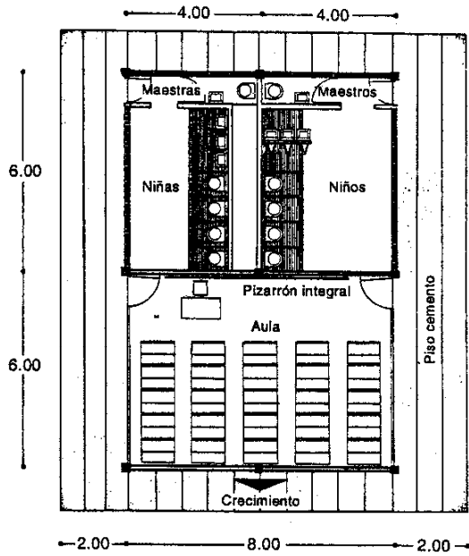
Aula tipo
