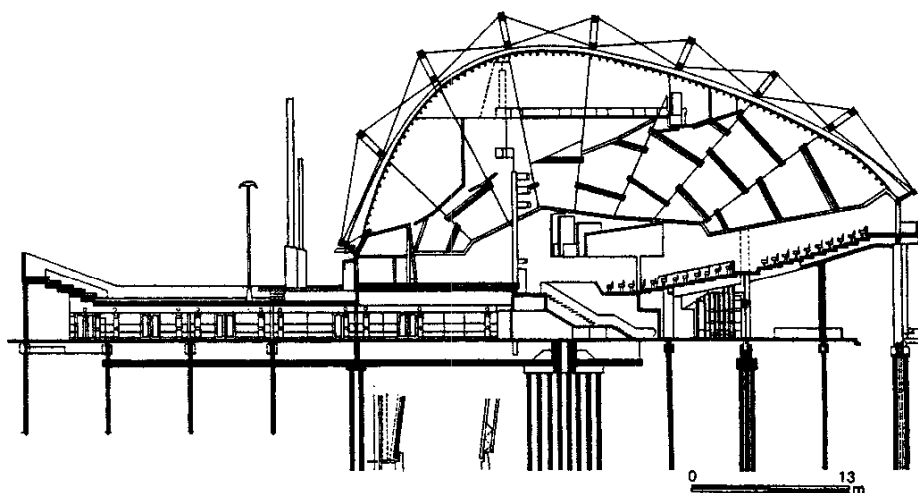
Corte longitudinal
