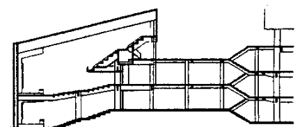
Corte longitudinal
