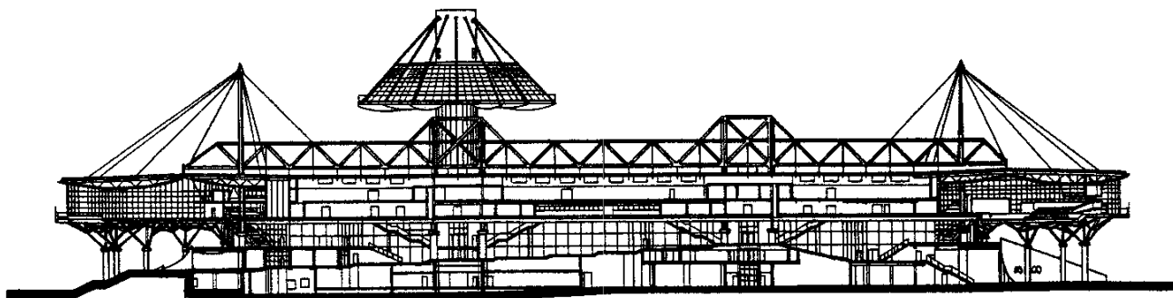
Corte longitudinal
