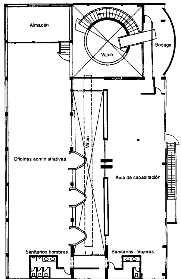
Planta alta
