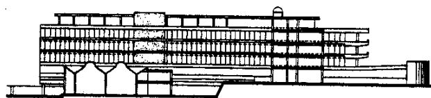
Corte longitudinal por aulas
