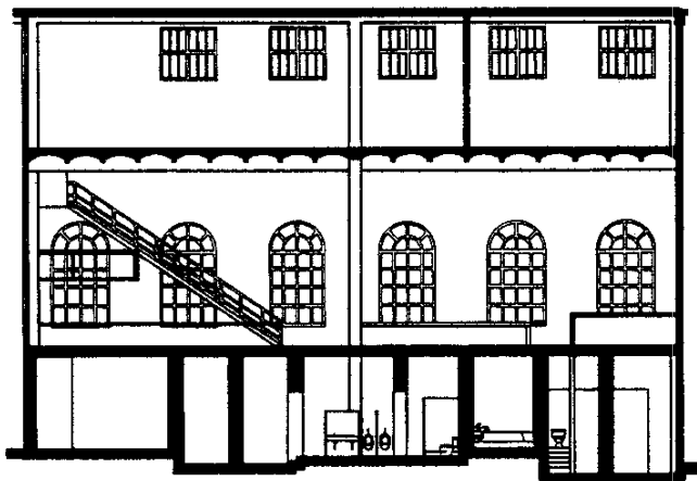
Corte B-B'
