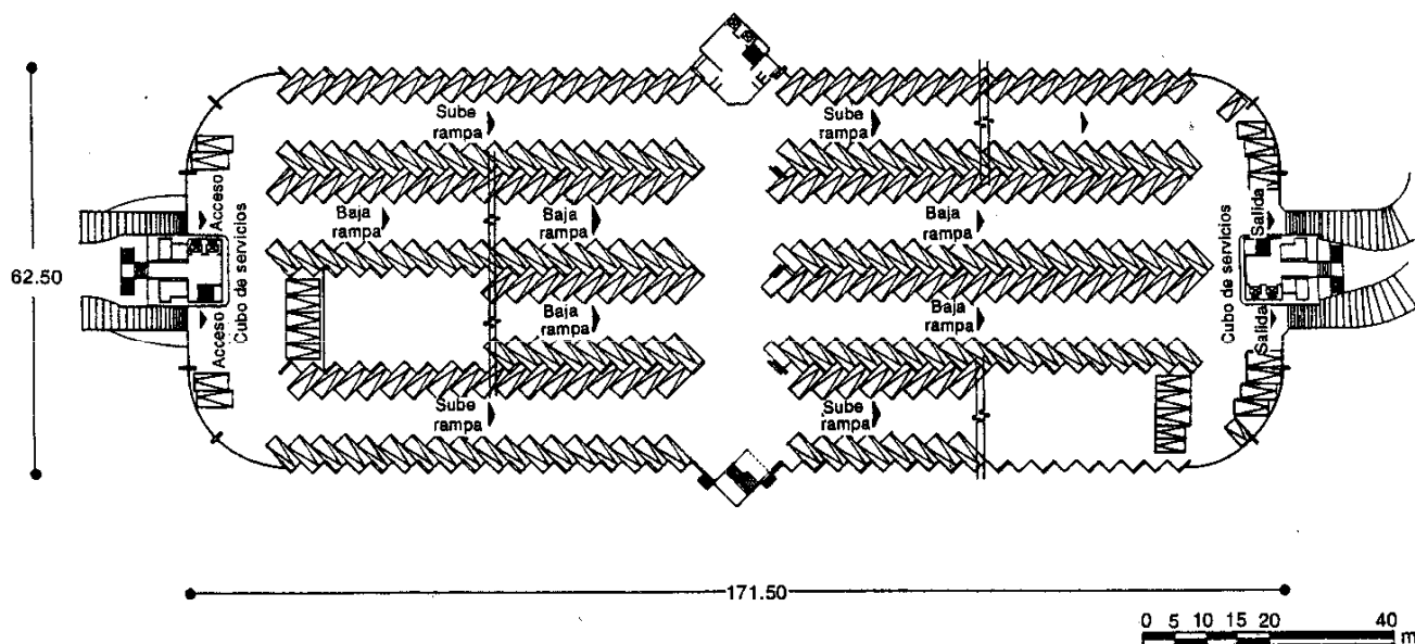
Planta
