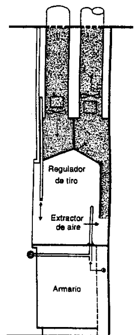
Corte
