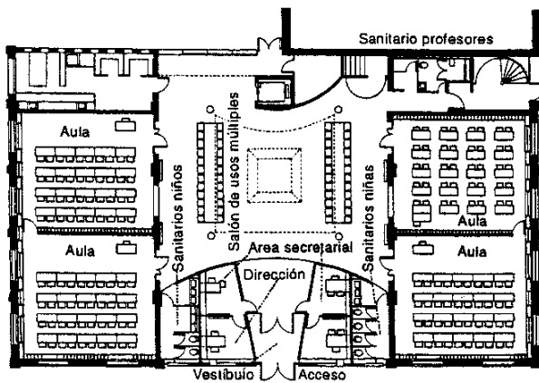
Planta baja
