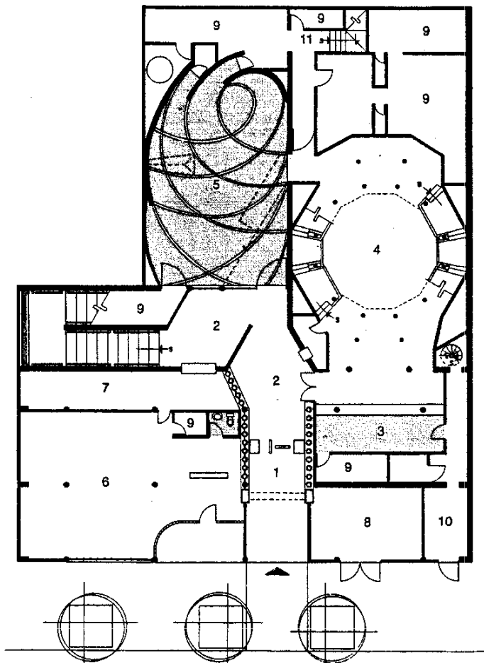
Planta baja
