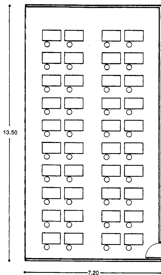
Taller de dibujo para 40 alumnos
