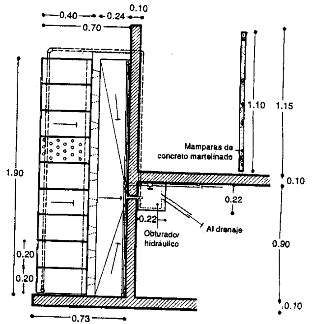
Detalle mingitorios
